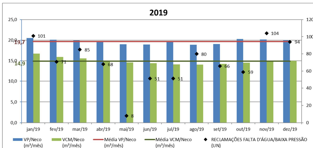
Gráfico 5: 2019 - VP/Neco e VCM/Neco e Médias Anuas (fonte: SISPERDAS) e Falta D'Água/Bx Pressão (fonte: ISODADOS)
