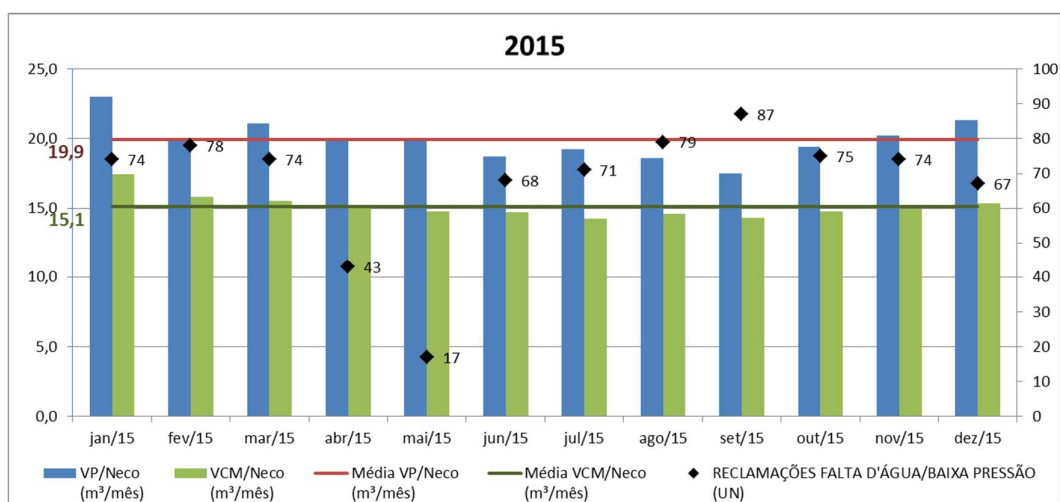
Gráfico 1: 2015 - VP/NEco e VCM/NEco e Médias Anuais (fonte: SISPERDAS) e Falta D'Água/Bx Pressão (fonte: ISODADOS)
