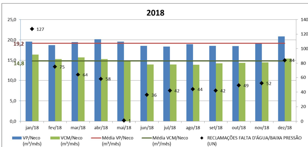
Gráfico 4: 2018 - VP/Neco e VCM/Neco e Médias Anuais (fonte: SISPERDAS) e Falta D'Água/Bx Pressão (fonte: ISODADOS)
