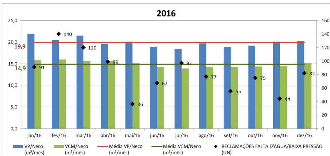
Gráfico 2: 2016 - VP/Neco e VCM/Neco e Médias Anuais (fonte: SISPERDAS) e Falta D'Água/Bx Pressão (fonte: ISODADOS)
