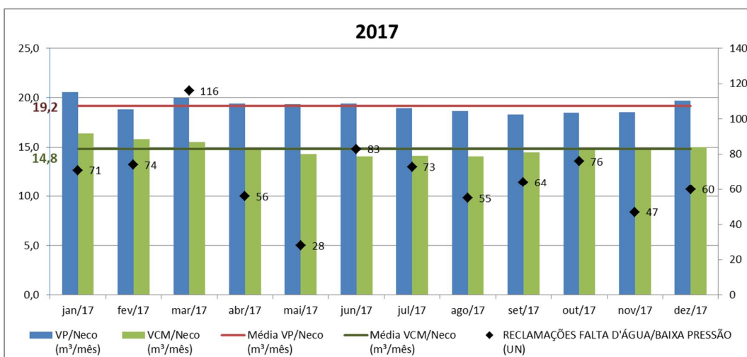
Gráfico 3: 2017 - VP/Neco e VCM/Neco e Médias Anuais (fonte: SISPERDAS) e Falta D'Água/Bx Pressão (fonte: ISODADOS)
