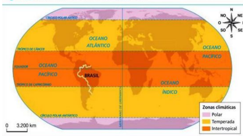
Figura 2. Mundo: zonas térmicas ou climáticas
