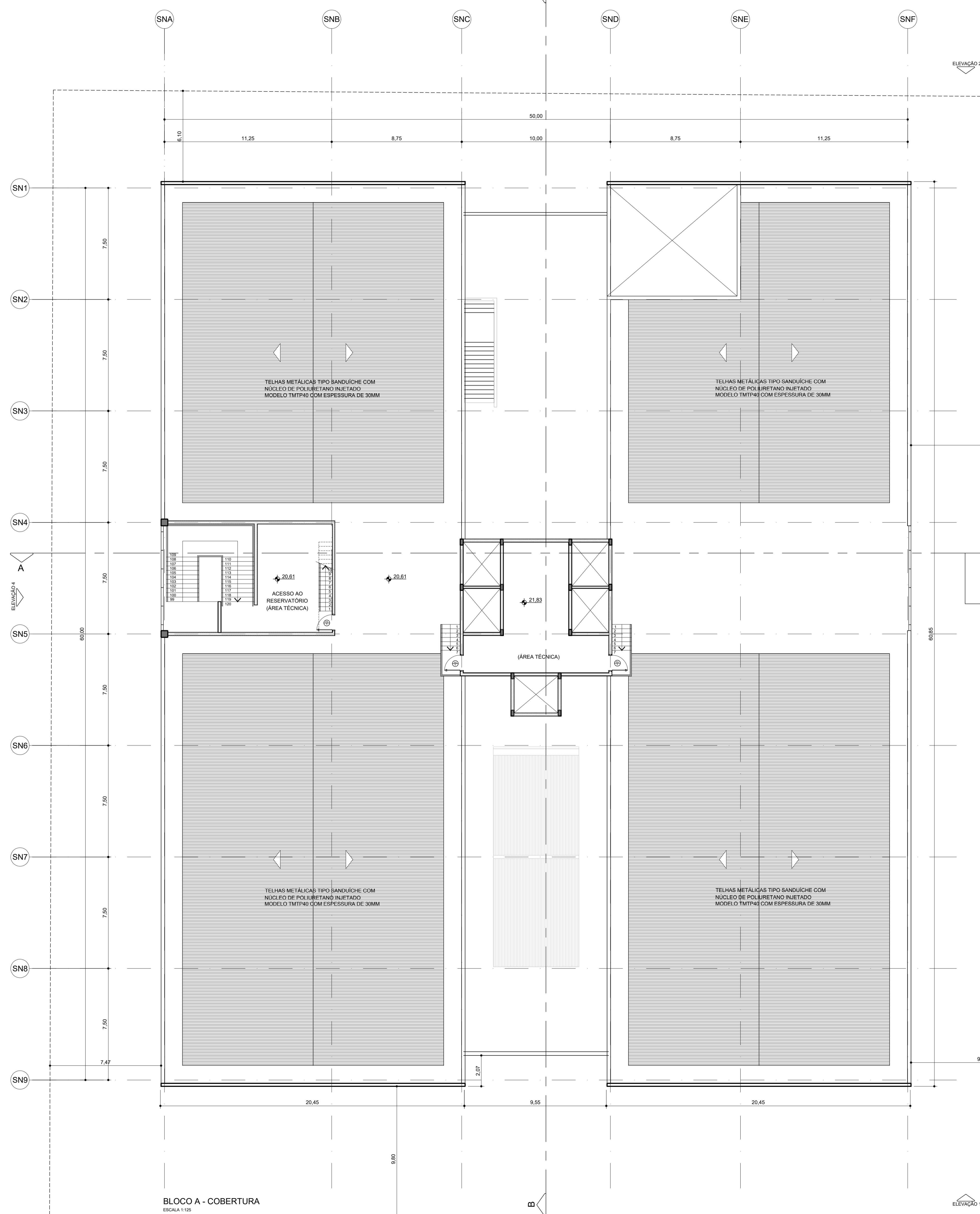
BLOCO A - COBERTURA ESCALA 1:125
