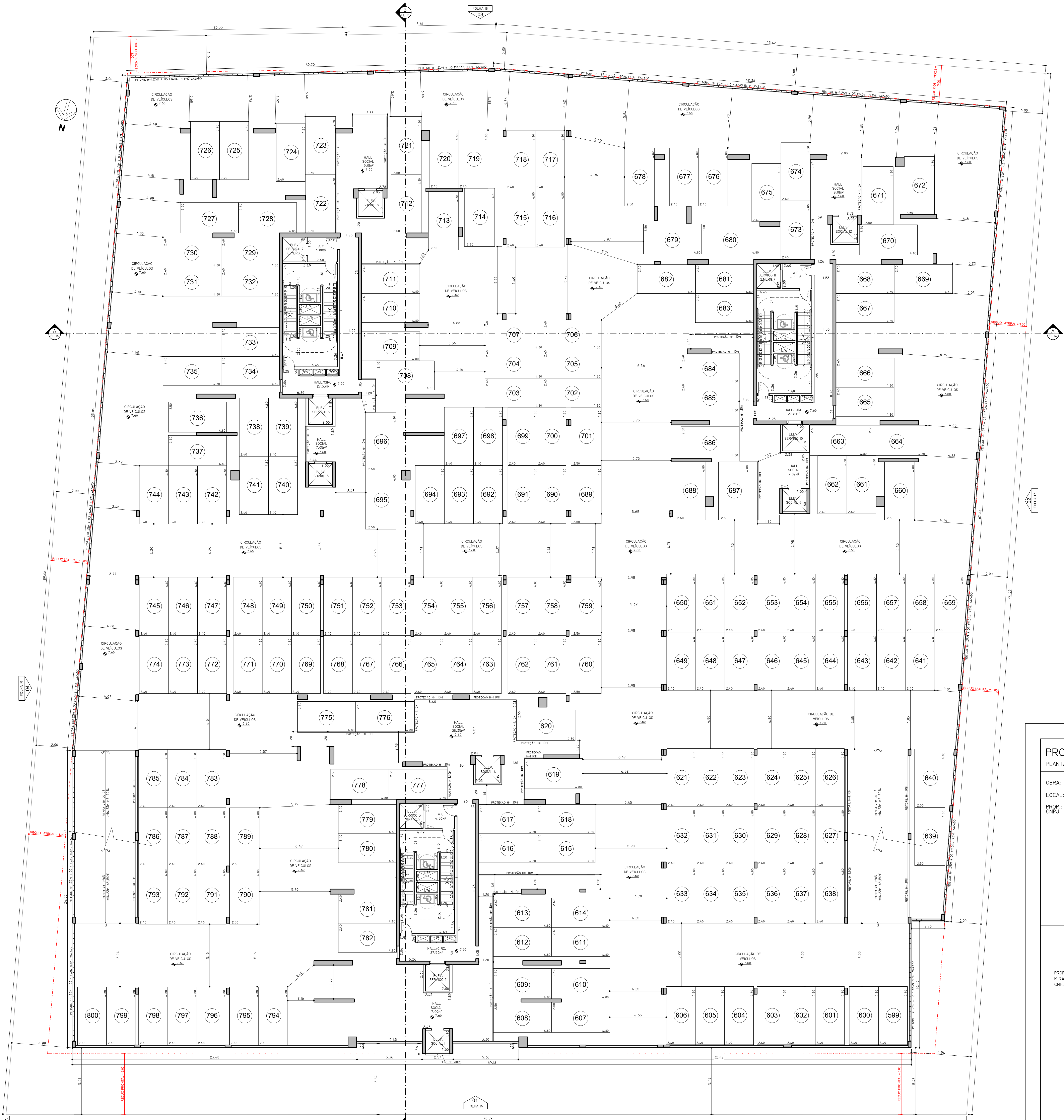
PLANTA MEZANINO G2 ESCALA: 1:125
