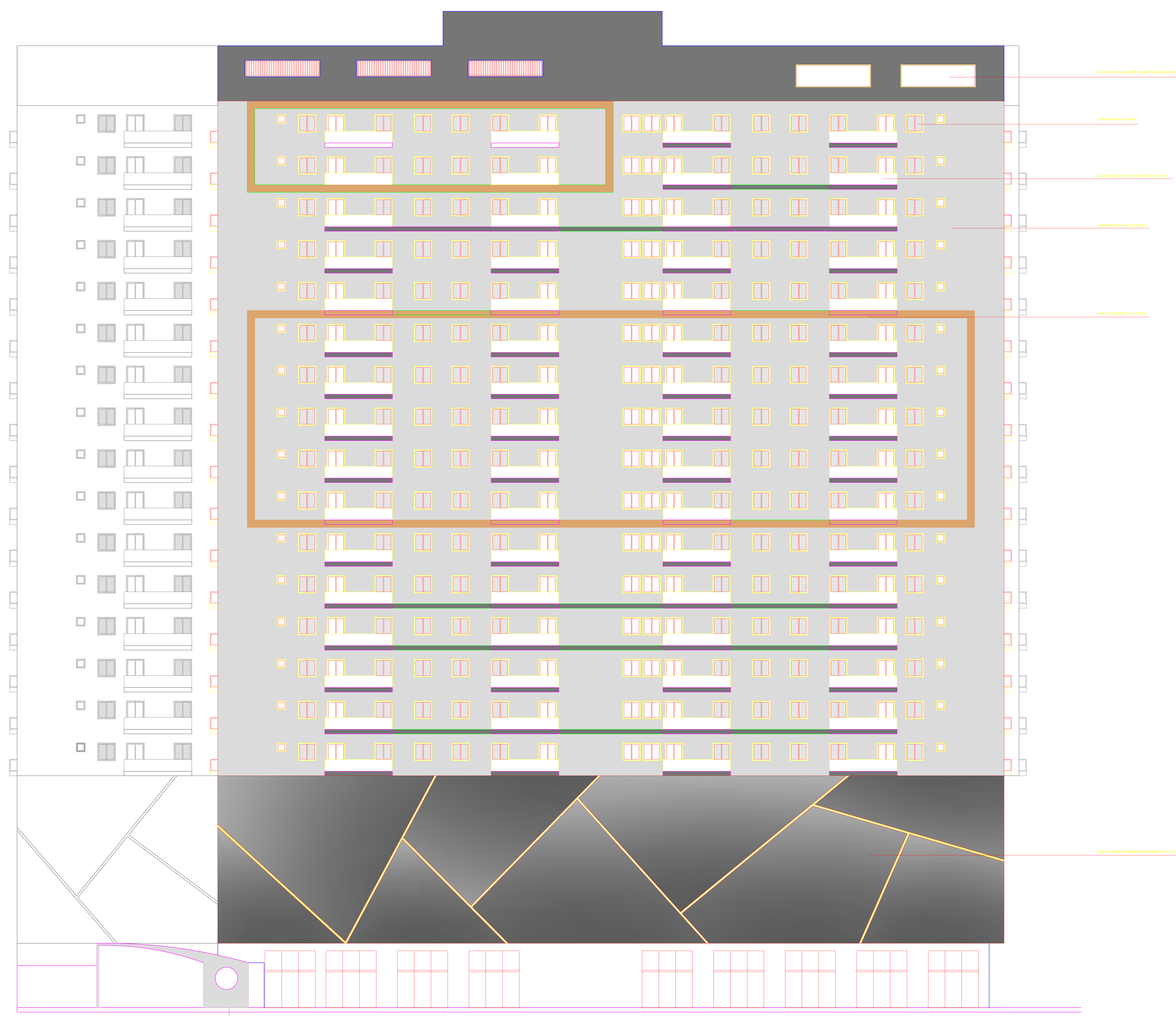
FACHADA 04 - RUA MARQUÊS DE HERVAL ESC. 1:100
