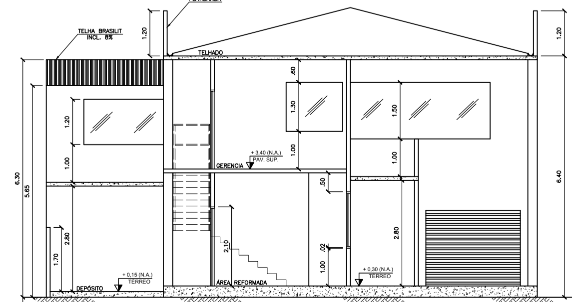
5 CORTE CD ESC.: 1:100
