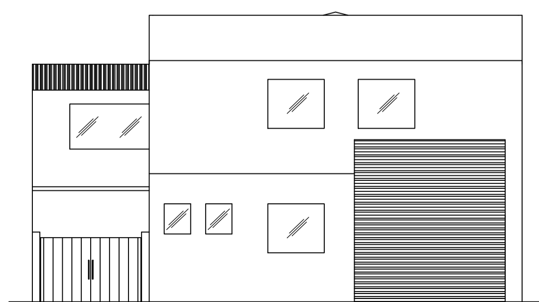
6 FACHADA 01 ESC.: 1:100
