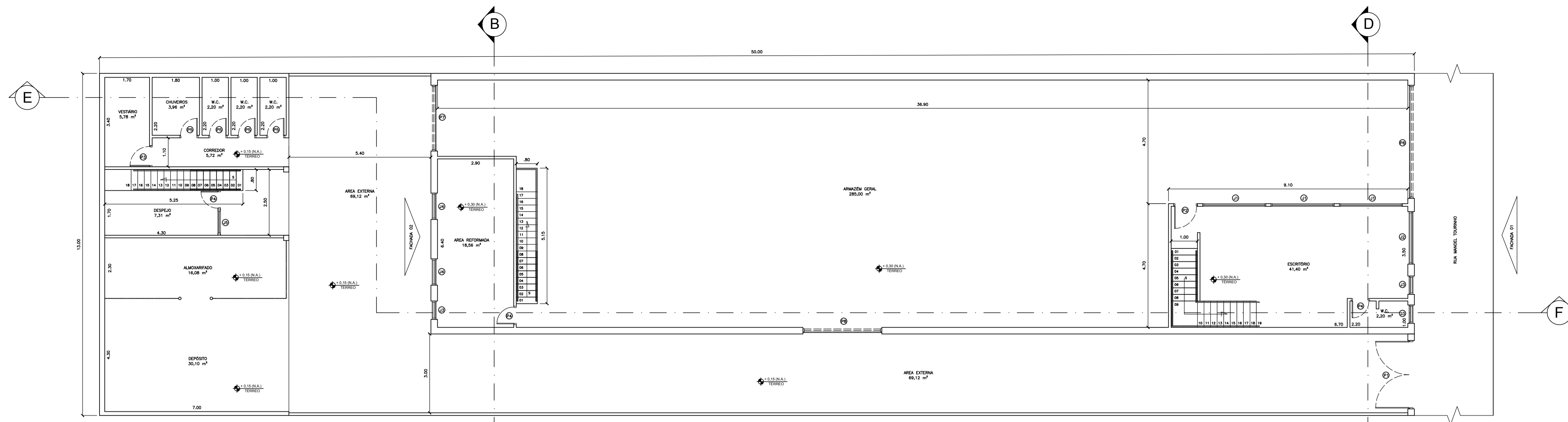
1 PLANTA PAV. TÉRREO ESC.: 1:100
