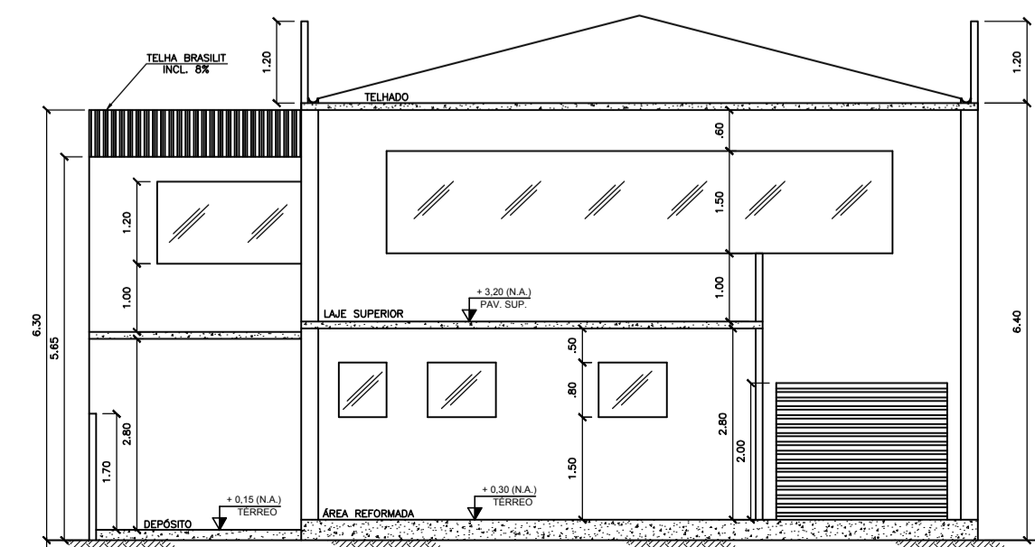
4 CORTE AB ESC.: 1:100
