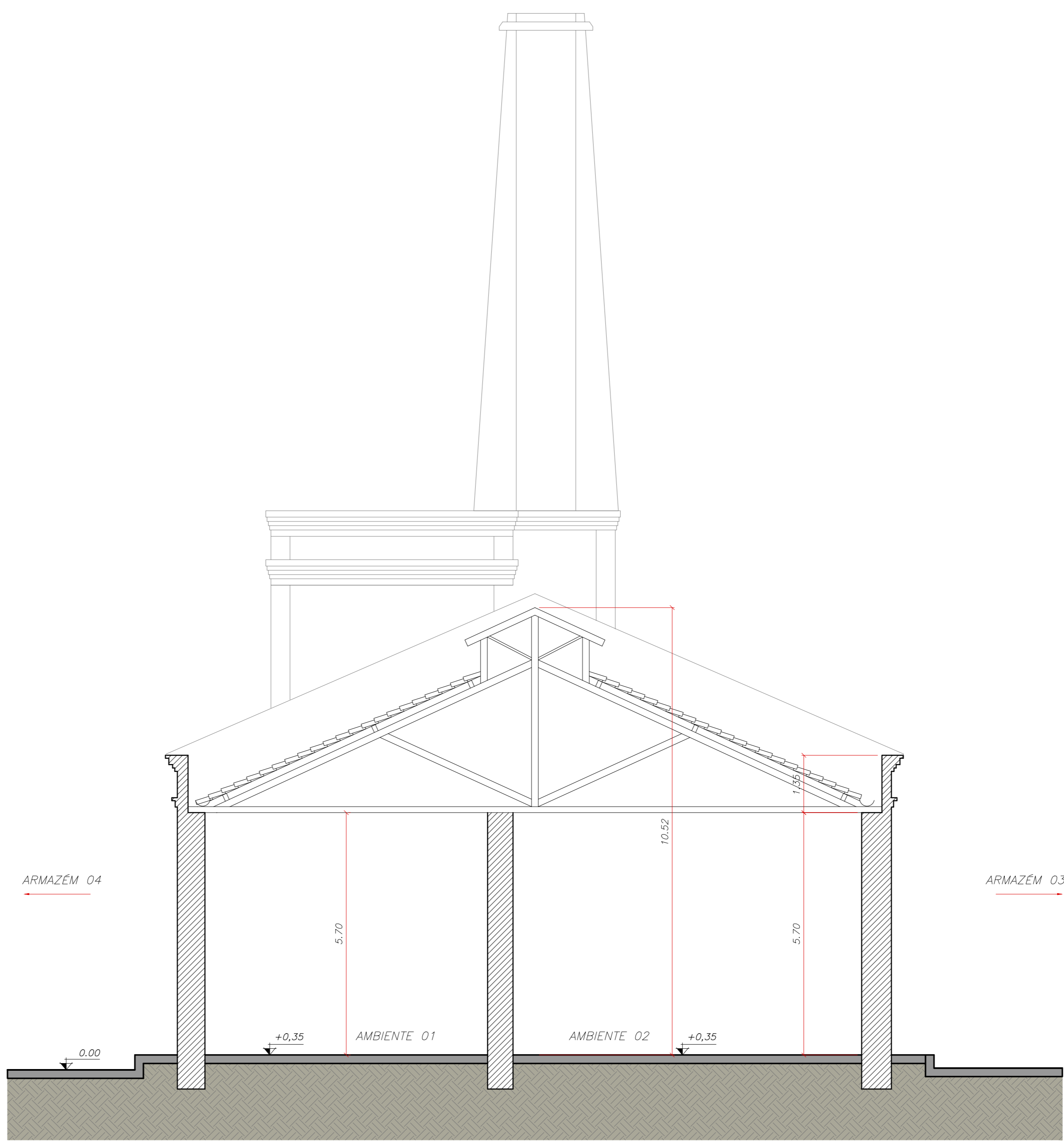
05 CORTE A-A - CASA DE PEDRA ESCALA 1/75
