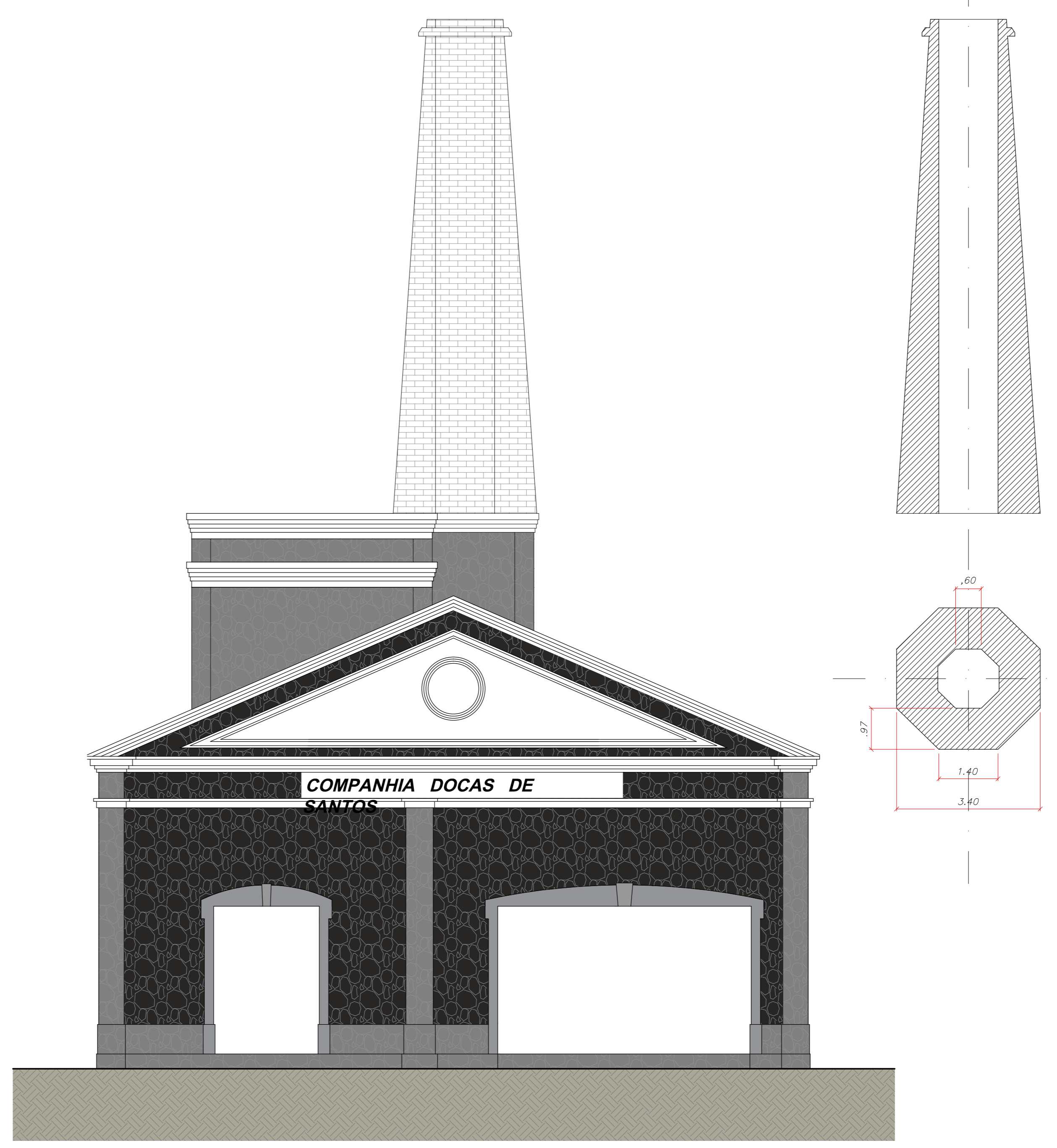
05 VISTA 01 - CASA DE PEDRA ESCALA 1/75
