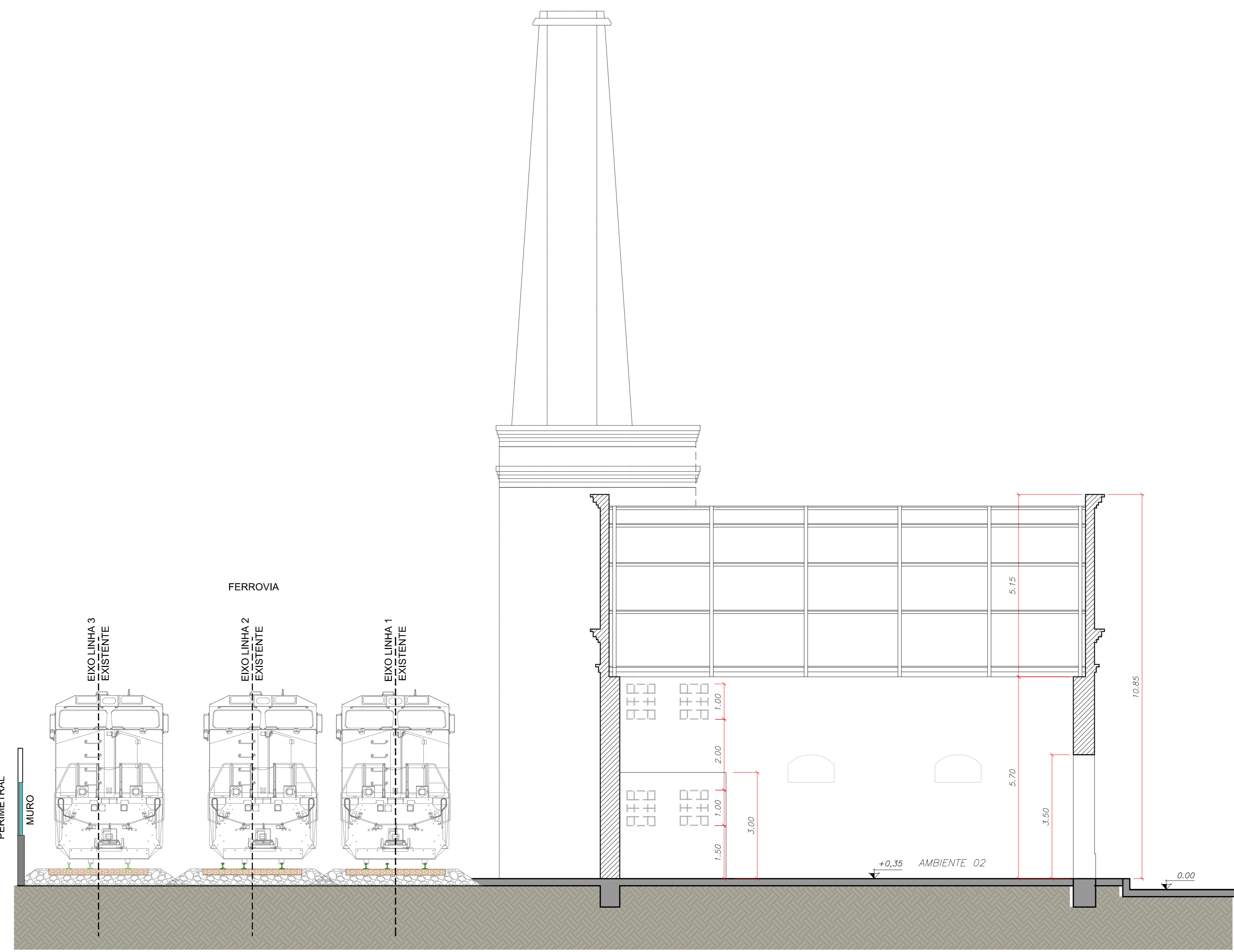
05 CORTE B-B - CASA DE PEDRA ESCALA 1/75
