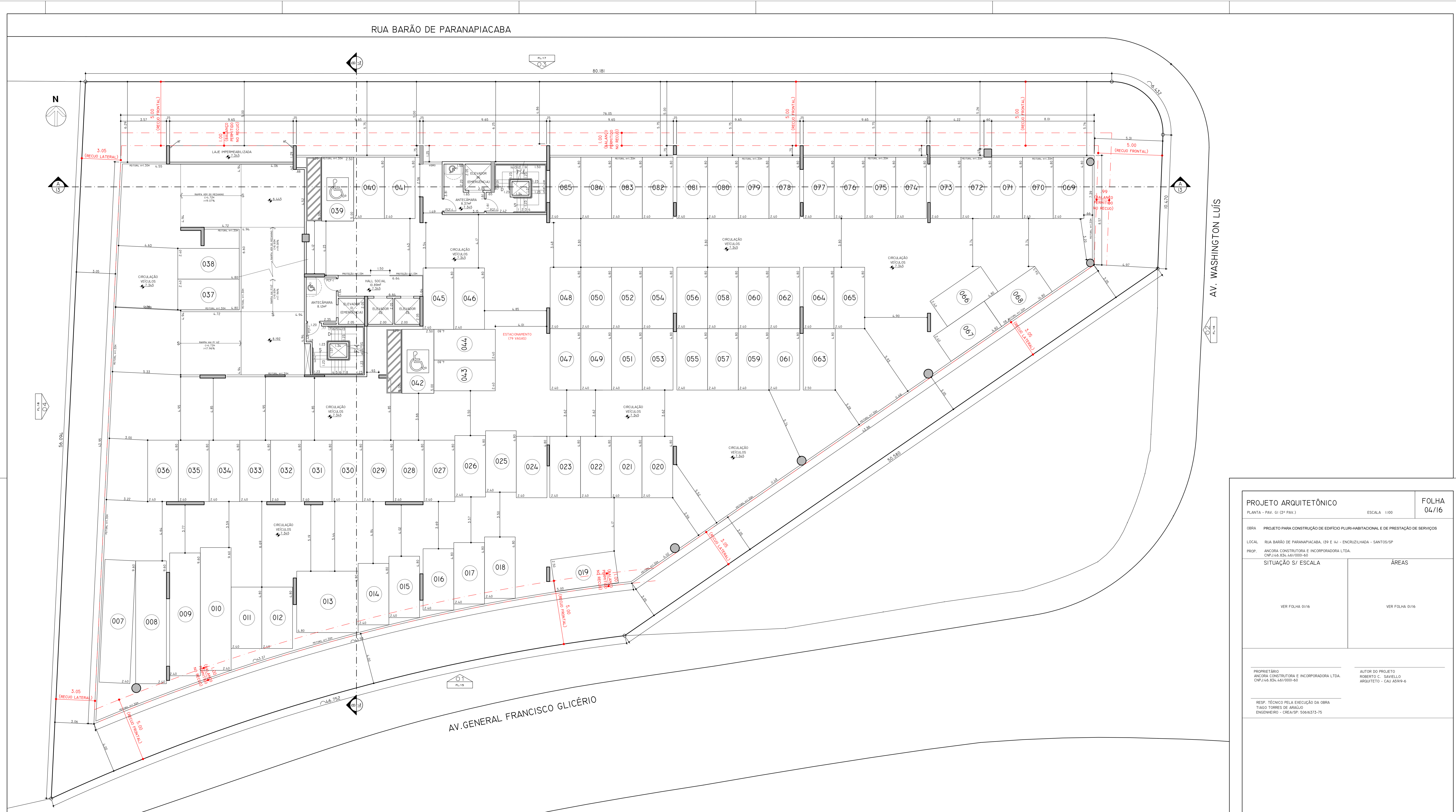
PLANTA PAV. GI (3º PAV.) ESCALA: 1:100
