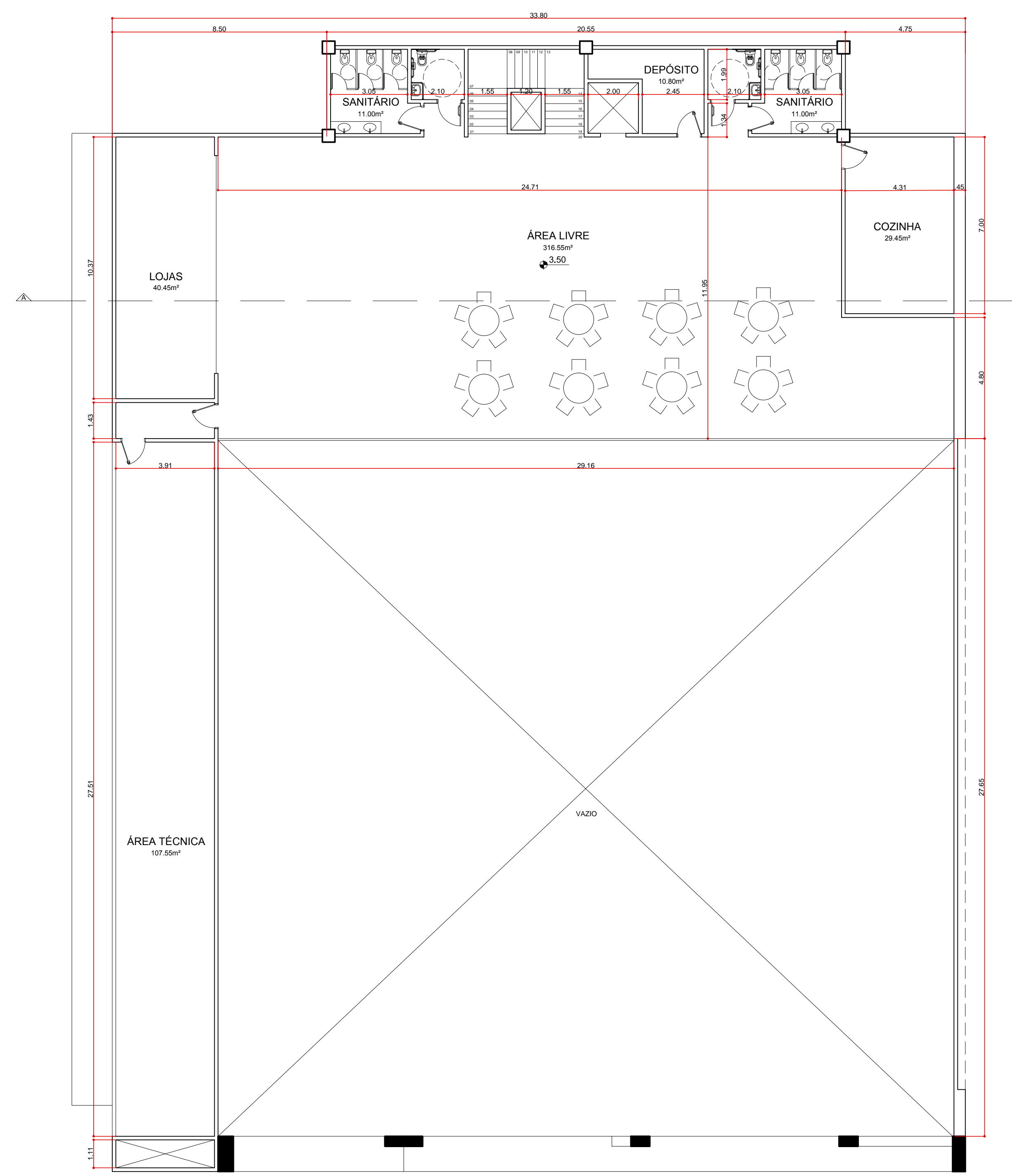
PLANTA MEZANINO esc. - 1:125
