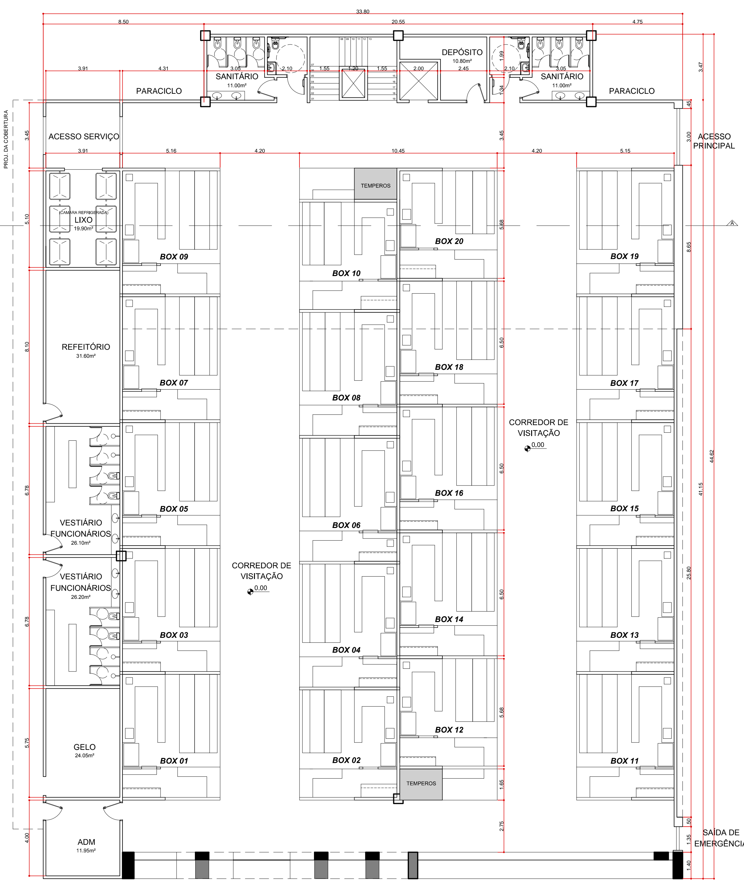
PLANTA TÉRREO esc. - 1:125
