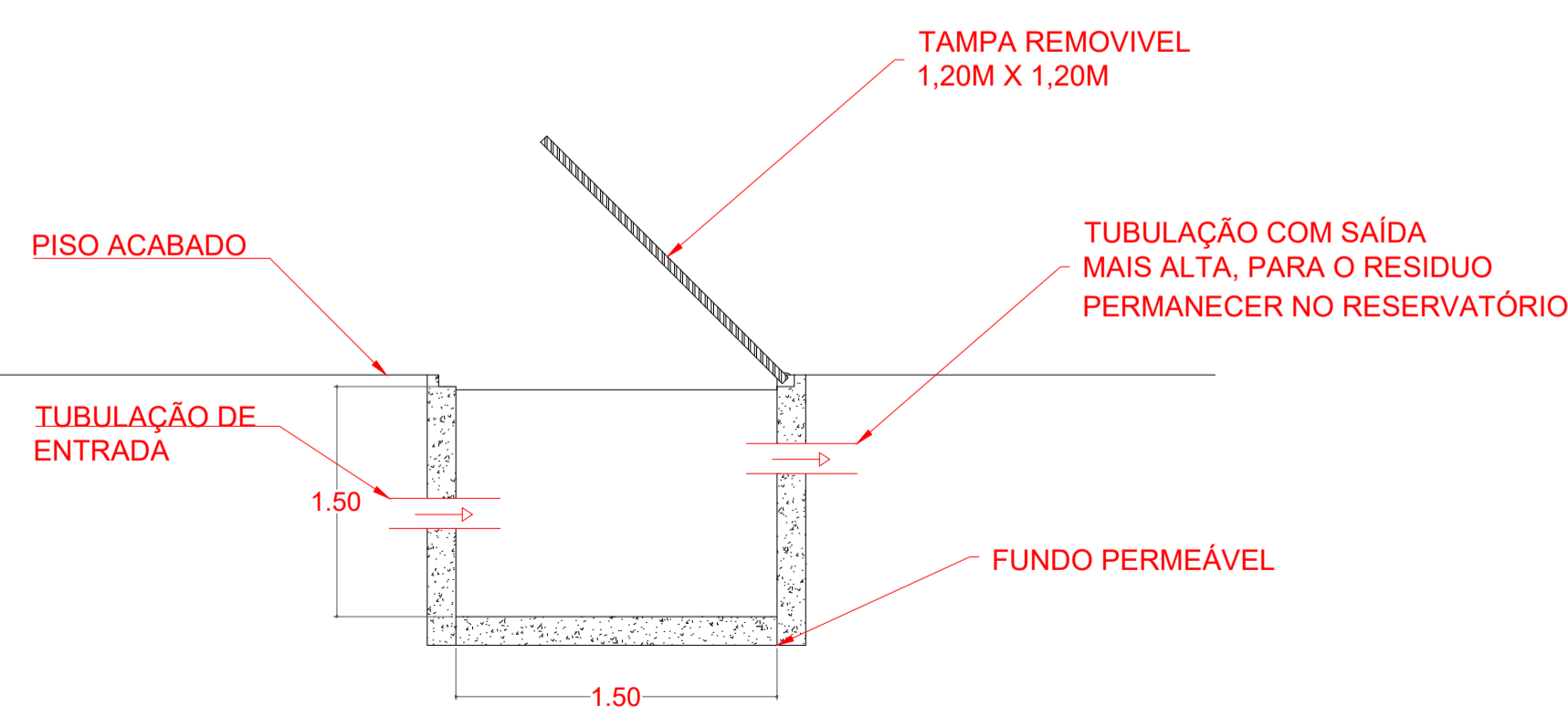
DETALHE: CAIXAS DE DRENAGEM DE  GUAS PLUVIAIS E SEGMENTA O DE RESIDUO S LIDO DO P TIO S/ ESCALA
