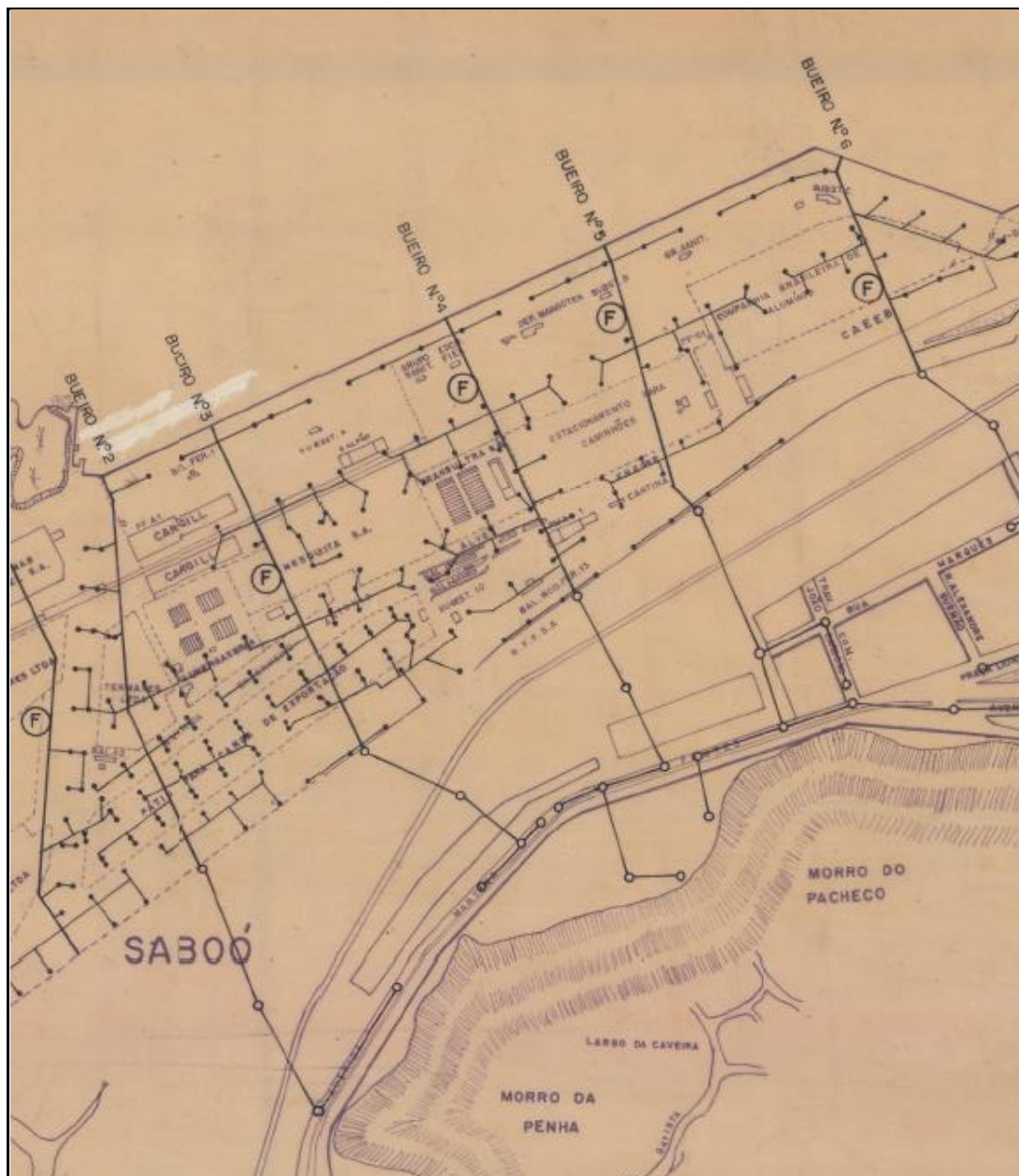
Figura 1 - Croqui da Bacia do Bueiro 04
