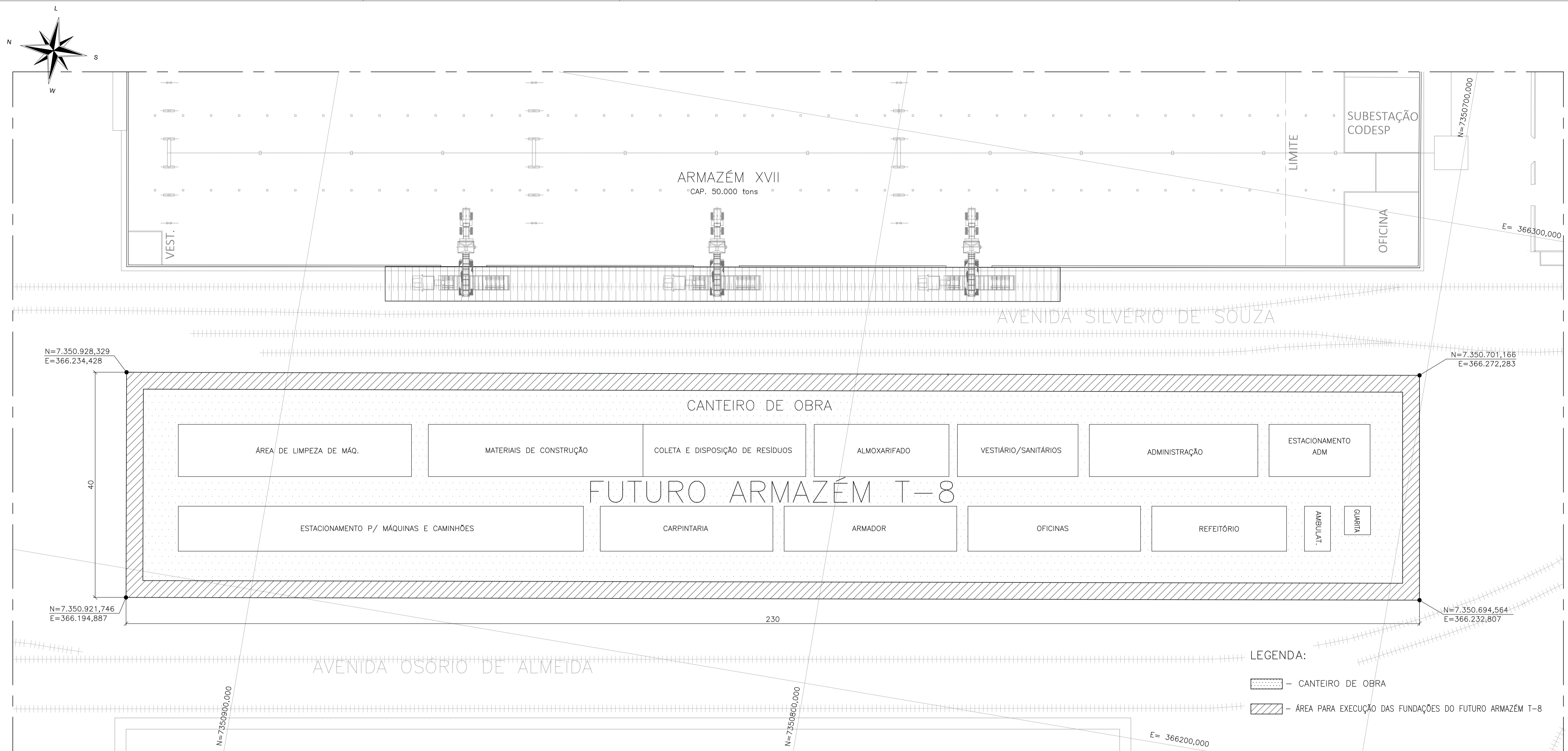
CANTEIRO DE OBRAS ESC. 1:350
