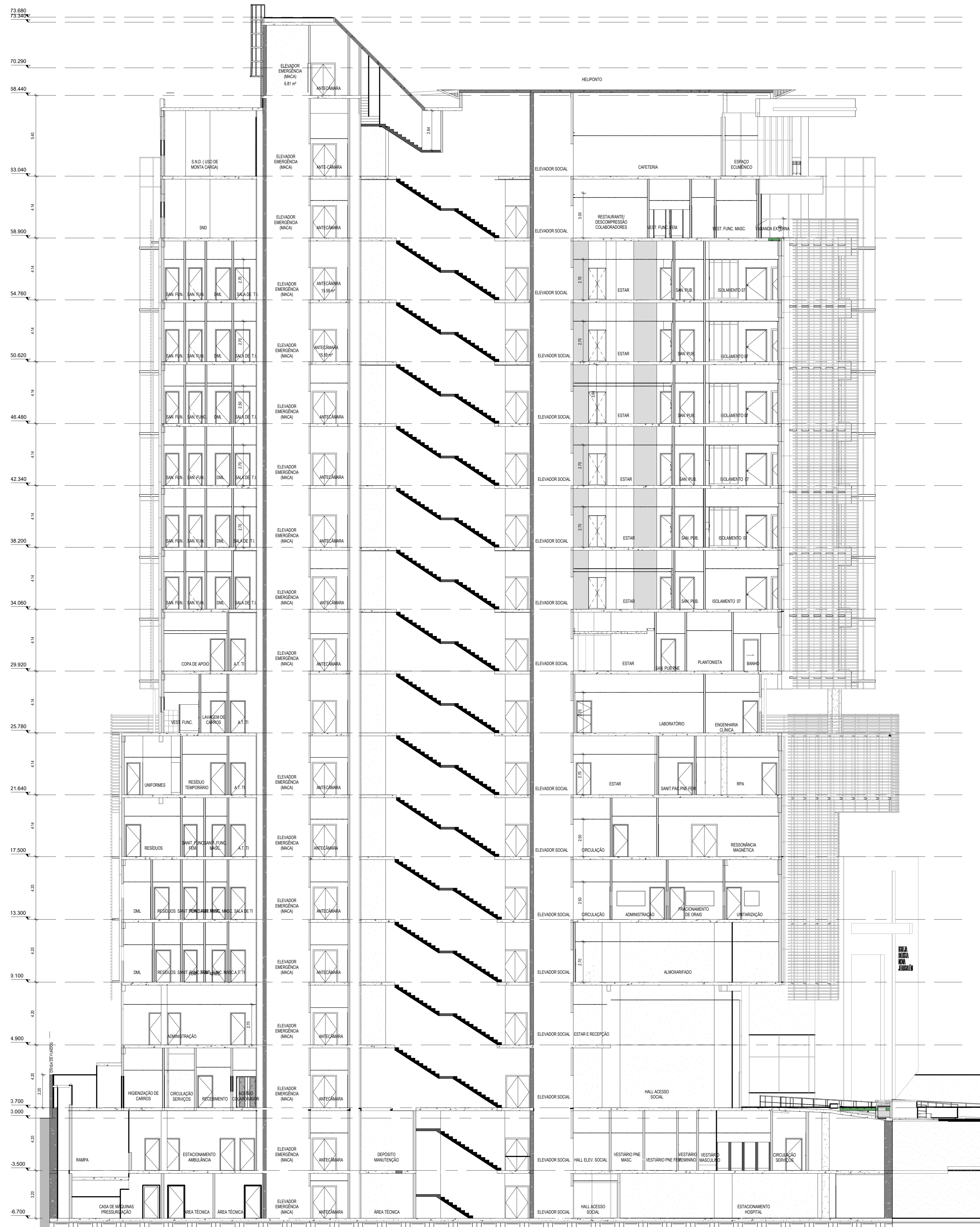
A CORTE AA 1:125
