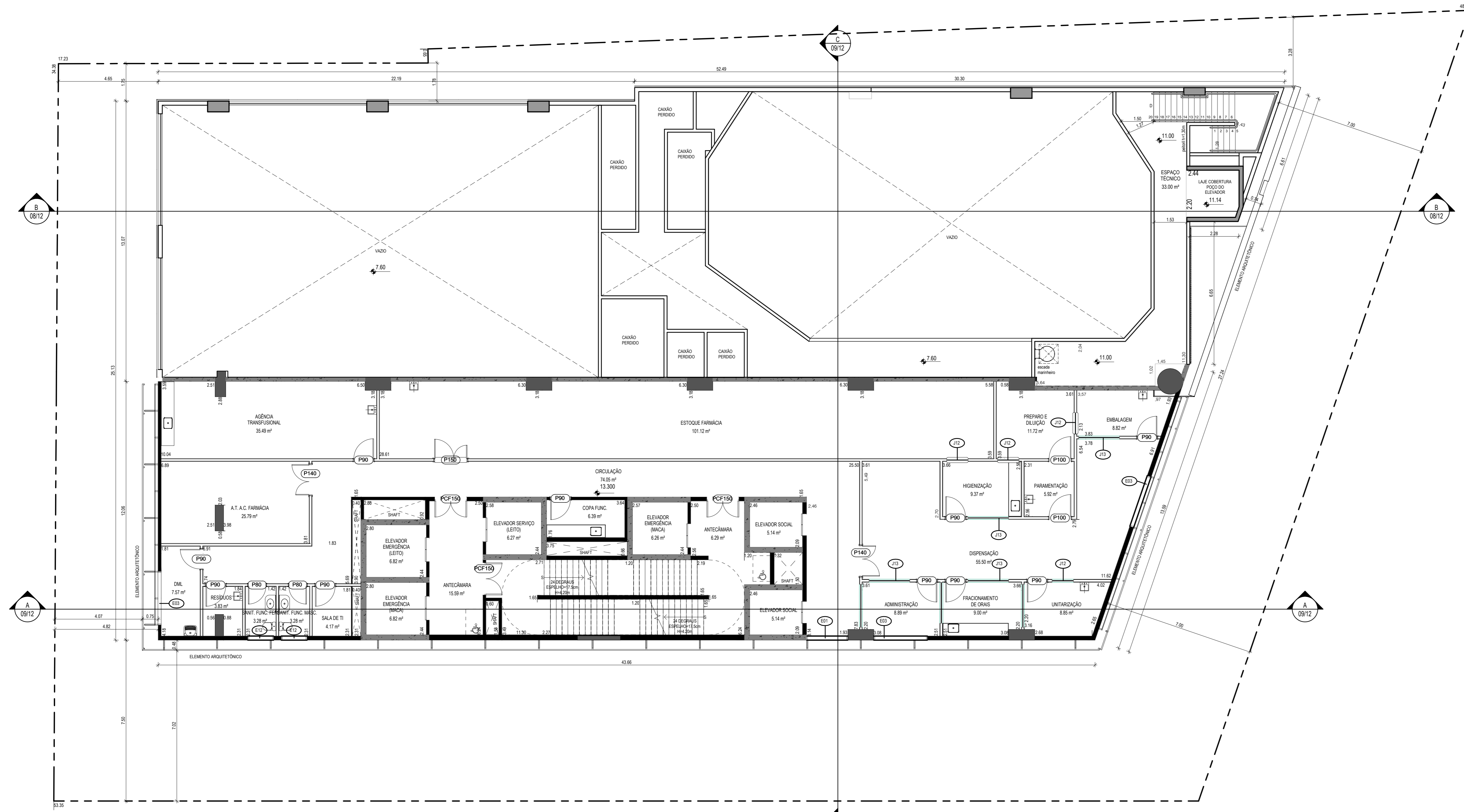
2 4º PAVIMENTO - FARMÁCIA CENTRAL, AG. TRANSFUSIONAL 1:100
